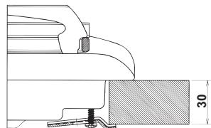
Монтаж крюка для опорных брусков H=30\text{mm}
