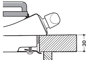
Position du crochet pour top H=30mm
