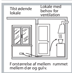
Eksempler på ventilationsåbninger for luft til forbrænding
