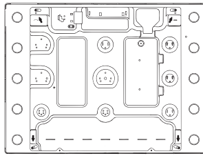
Posição do gancho para H=30mm
