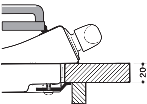
Position du crochet pour top H=20mm
