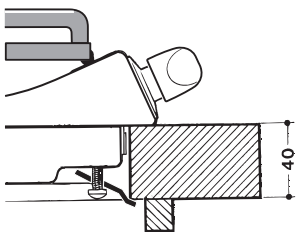
Stand haak voor keukenblad H=40mm
