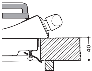
Placering af krog ved topstykke H=40mm
