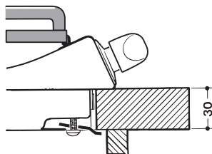
Position der Haken für Arbeitsplatten H=30mm
