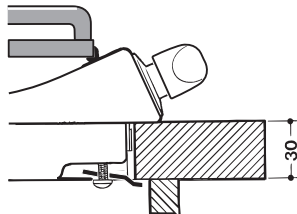
Stand haak voor keukenblad H=30mm
