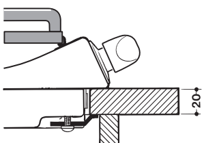
Position der Haken für Arbeitsplatten H=20mm
