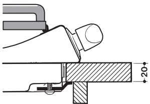
Posición del gancho para superficies H=20mm
