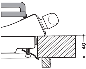
Posição do gancho para H=40mm
