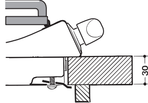
Placering af krog ved topstykke H=30mm
