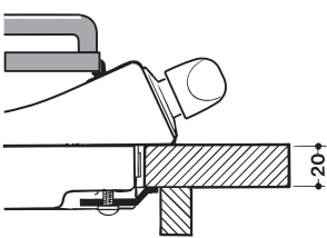
Posição do gancho para H=20mm
