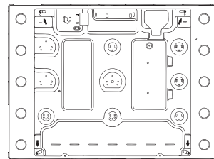
Placering af krog ved topstykke H=30mm
