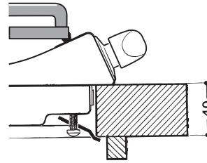
Position du crochet pour top H=40mm
