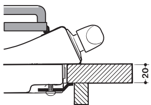
Placering af krog ved topstykke H=20mm
