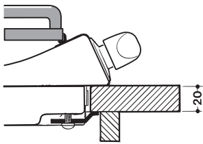
Posizione gancio per top H=20mm
