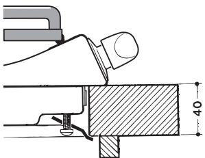
Position der Haken für Arbeitsplatten H=40mm
