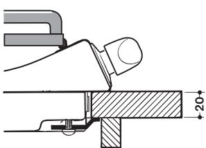
Stand haak voor keukenblad H=20mm
