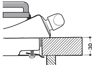
Posizione gancio per top H=30mm
