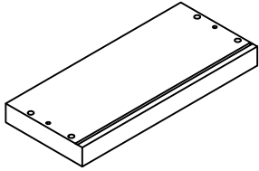
1 Top x1 (32cm x 14cm)
